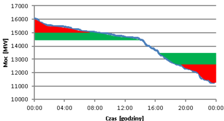
Rys. 15. Uszeregowany przebieg mocy KSE w dniu 7.07.2013 z naniesionymi obszarami przesunięcia zapotrzebowania na moc.
