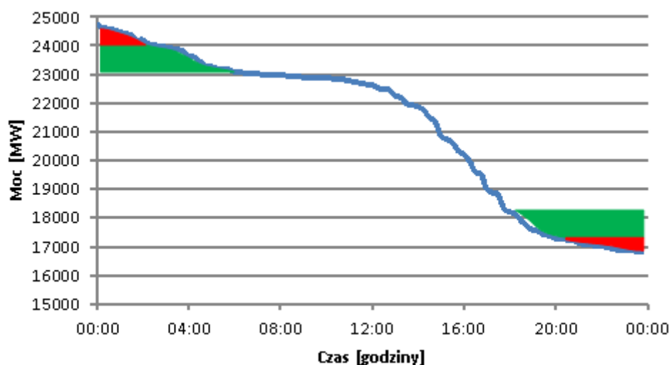
Rys. 11. Uszeregowany przebieg mocy KSE w dniu 10.12.2013 z naniesionymi obszarami przesunięcia zapotrzebowania na moc.
