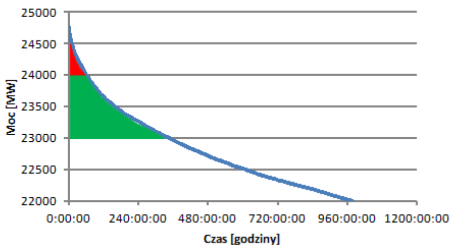
Rys. 9. Uszeregowany przebieg mocy KSE w 2013r. z naniesionymi obszarami przesunięcia zapotrzebowania na moc. Powiększenie zakresu powyżej 22000 MW.
