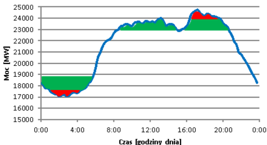
Rys. 12. Zapotrzebowanie mocy KSE w dniu 23.01.2013r. z naniesionymi obszarami przesunięcia zapotrzebowania na moc.
