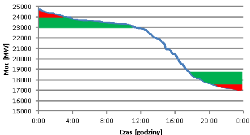
Rys. 13. Uszeregowany przebieg mocy KSE w dniu 23.01.2013 z naniesionymi obszarami przesunięcia zapotrzebowania na moc.
