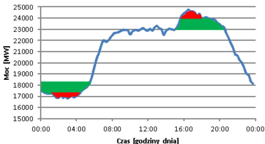
Rys. 10. Zapotrzebowanie mocy KSE w dniu 10.12.2013r. z naniesionymi obszarami przesunięcia zapotrzebowania na moc (dzień 1).
