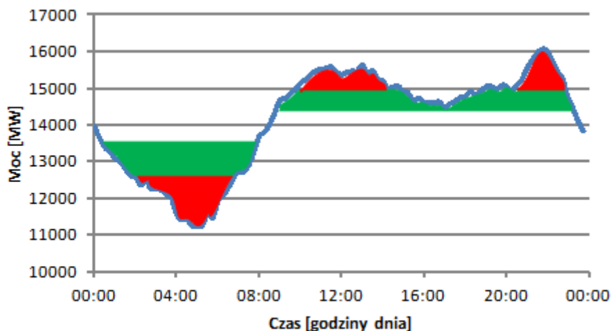
Rys. 14. Zapotrzebowanie mocy KSE w dniu 7.07.2013r. z naniesionymi obszarami przesunięcia zapotrzebowania na moc.
